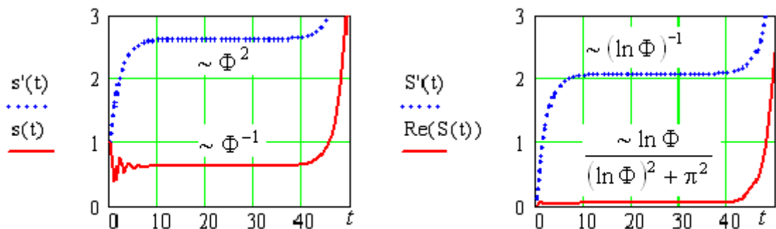
Рис. 3. Интегральные характеристики системы с возникновением бифуркации
