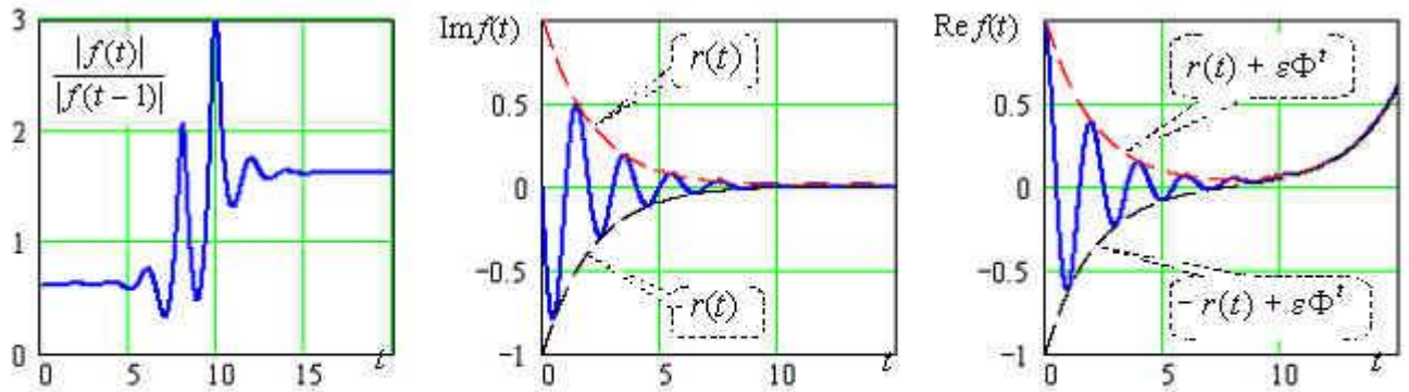
Рис. 1. Примерное развитие процесса f(t) = (-\Phi)^{-t} + \delta F(t)
