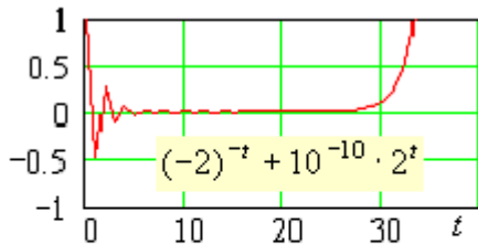
Рис. 4. Пример развития процесса, не имеющего дискретно-аддитивной рекурсии
